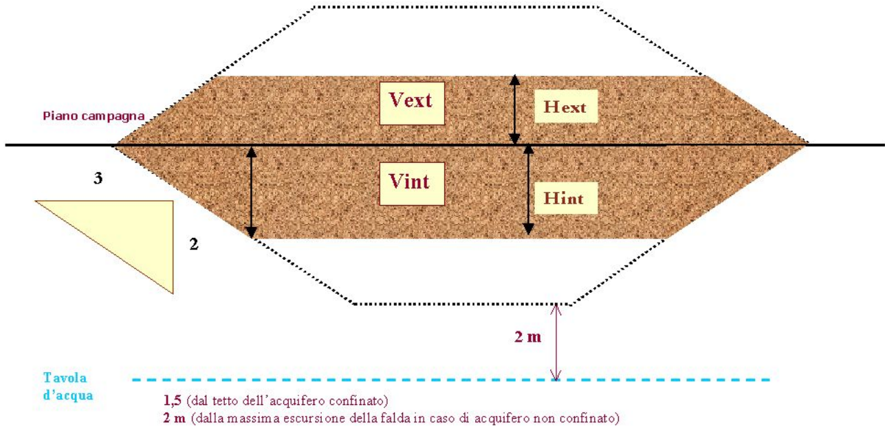
Fig. 10-14 – Schema semplificato di discarica in parte in scavo e in parte in rilevato
